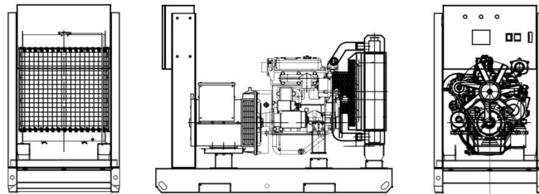
GPC35-6 (Abierta)
